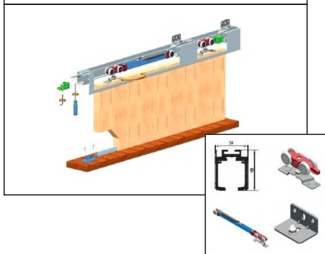
Sisteme culisante 9700
